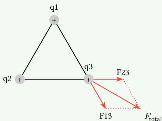
图 3. 位于等边三角形三个顶点处的电荷
