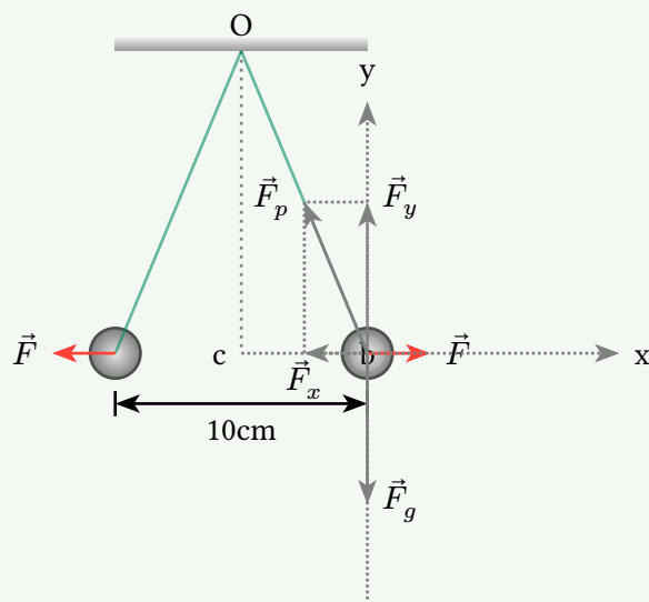
图 5. 悬挂在绝缘细线上的带电小球
