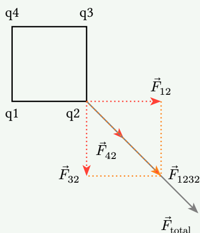
图 4. 位于正方形四个顶点处的电荷
