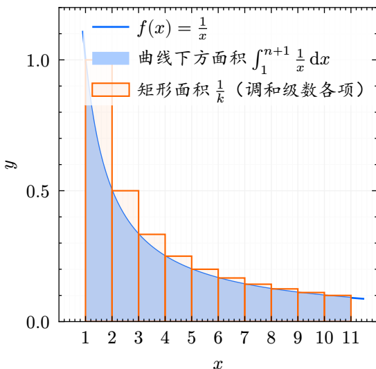
图1 积分判别法示意
