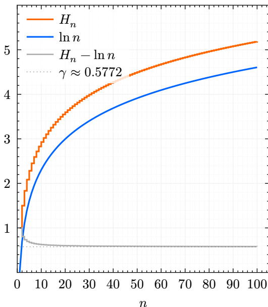
图2 调和数 H_n 、对数函数 \ln n 及其差值 H_n - \ln n 随 n 的变化趋势。
