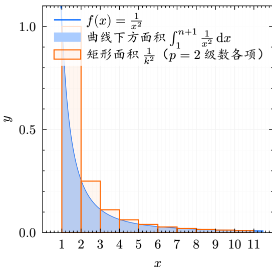
图3 p = 2 时积分判别法示意
