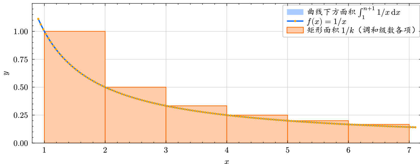
图1 积分判别法示意：蓝色曲线为 f(x) = 1/x ，橙色矩形代表调和级数前6项（高度 1/k 、宽度1，左端位于 x = k 处）。由于 f(x) 单调递减，在区间 [k, k+1] 上恒有 1/k \geq 1/x ，因此每个矩形面积均大于其下方曲边梯形的面积，求和即得 H_n > \int_1^{n+1} 1/x \, dx = \ln(n+1) ，从而推出调和级数发散。
