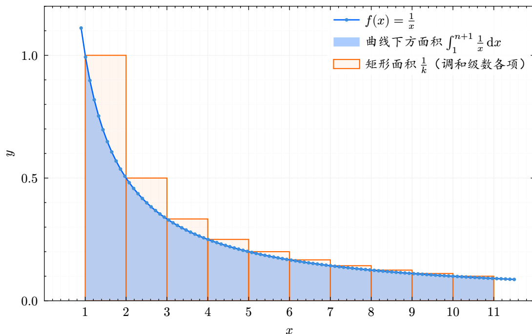
图 1 积分判别法示意
