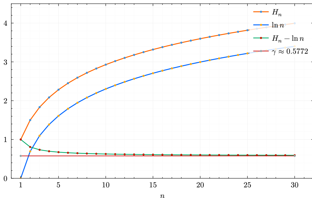
图2 调和数 H_n 、对数函数 \ln n 及其差值 H_n - \ln n 随 n 的变化趋势。可见 H_n 与 \ln n 均随 n 增大而增长，但二者之差逐渐趋近于欧拉—马歇罗尼常数 \gamma 。
