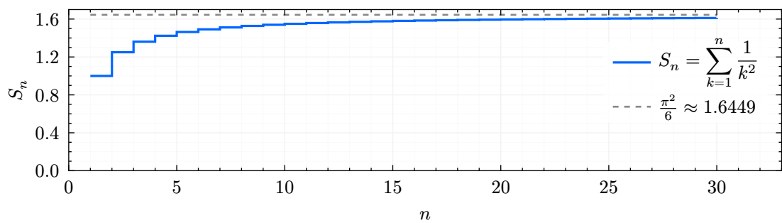
图 4 p = 2 时，部分和 S_n = \sum_{k=1}^n \frac{1}{k^2} 的收敛趋势。灰色虚线为极限值 \frac{\pi^2}{6} 。
