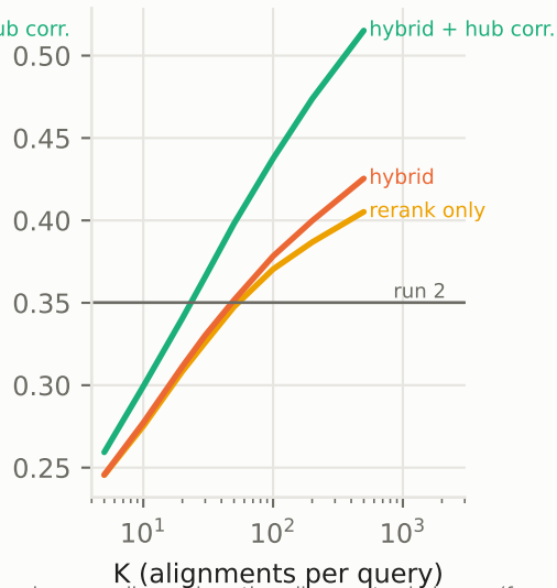
Hit@1
