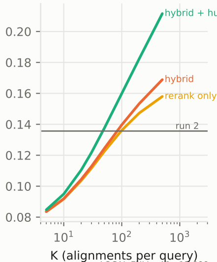
MAP
