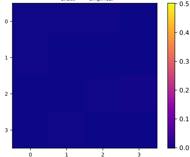
P_{\text{exact}} - P_{\text{empirical}}
