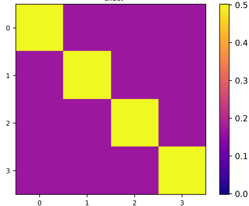
P_{\text{exact}}
