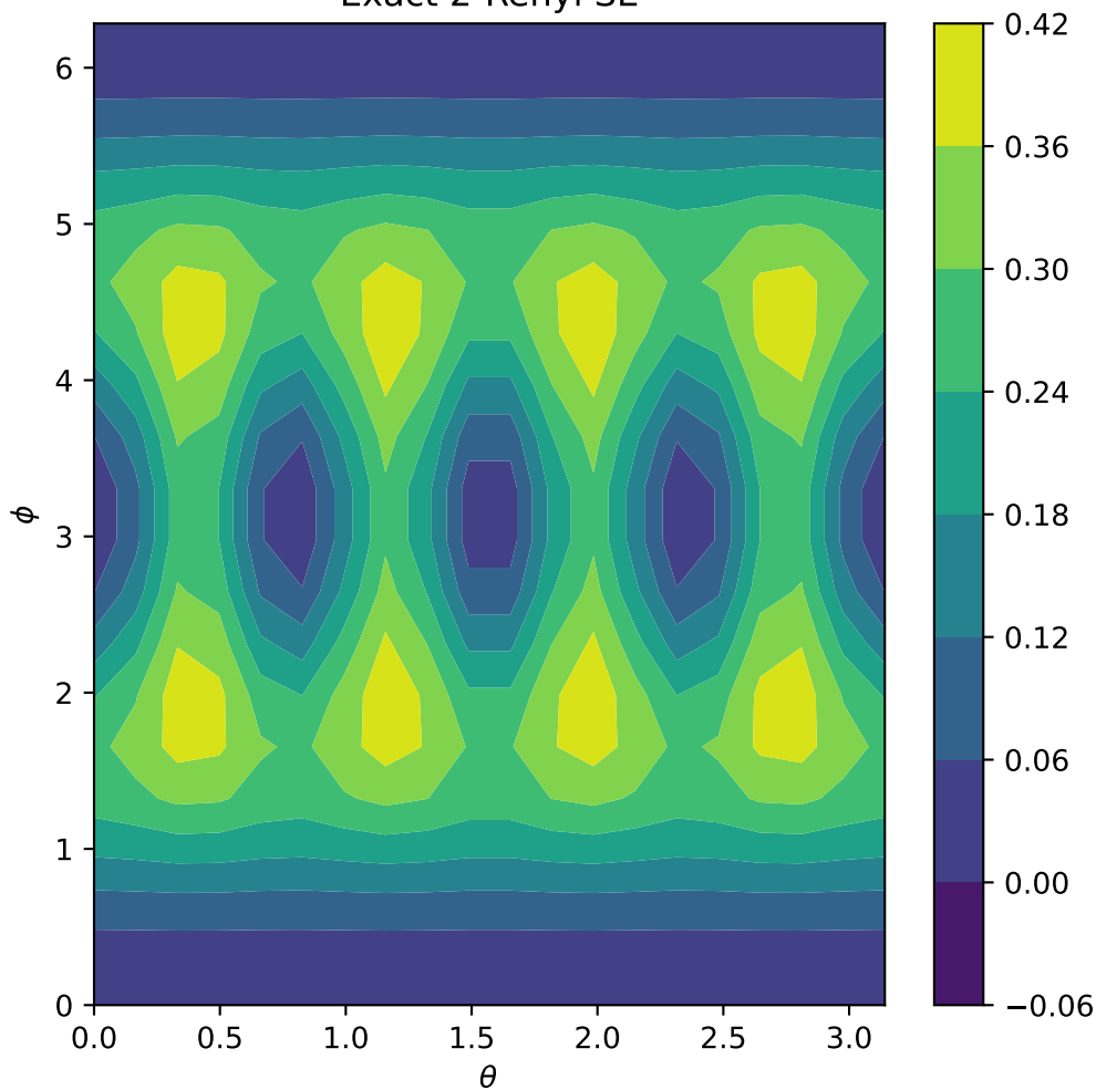
Exact 2-Renyi SE
