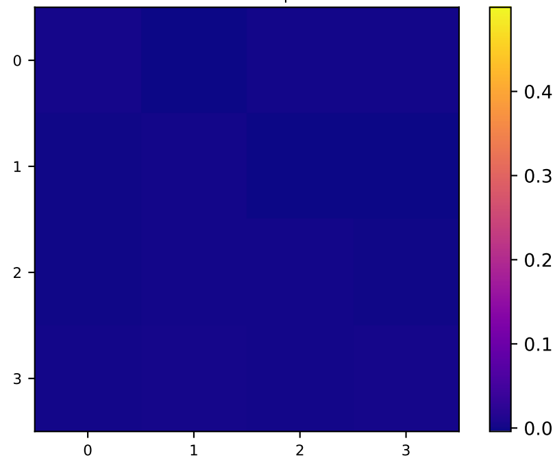
P_{\text{exact}} - P_{\text{empirical}}
