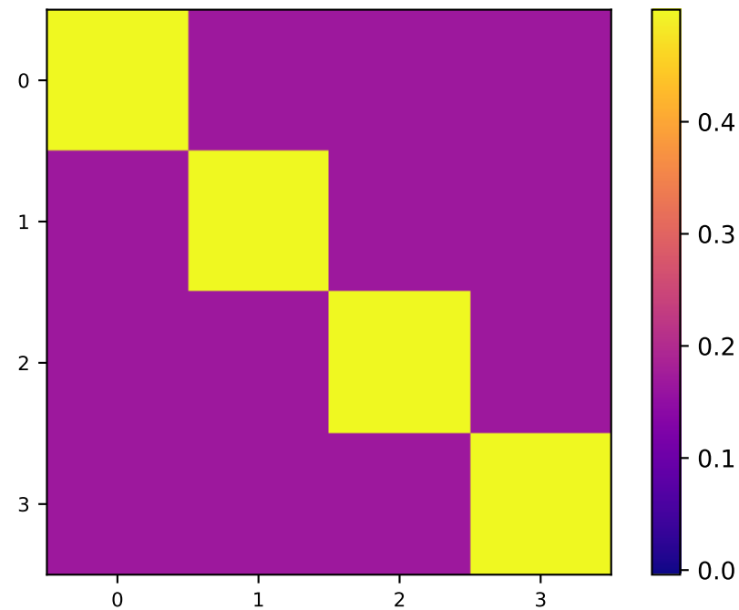
P_{\text{exact}}
