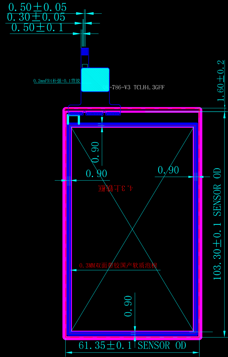
背视图
