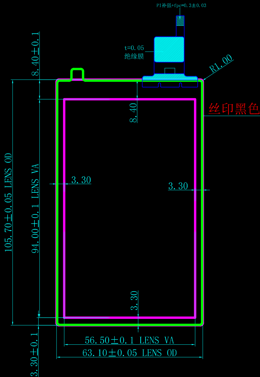
正视图
