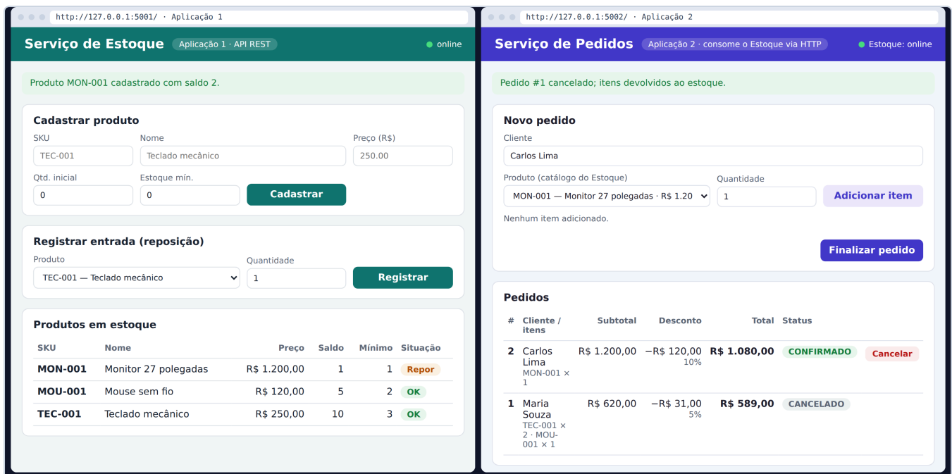
Figura 8: Pedido #1 cancelado: os itens voltaram ao Estoque (Teclado 10, Mouse 5).
