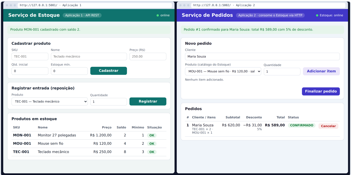
Figura 5: Pedido de R$ 620,00 confirmado com 5% de desconto. O Estoque baixou 2 teclados e 1 mouse.
