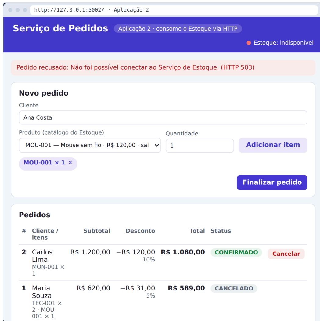
Figura 9: Com o Estoque desligado, o Pedidos indica a indisponibilidade e recusa o pedido com HTTP 503.
