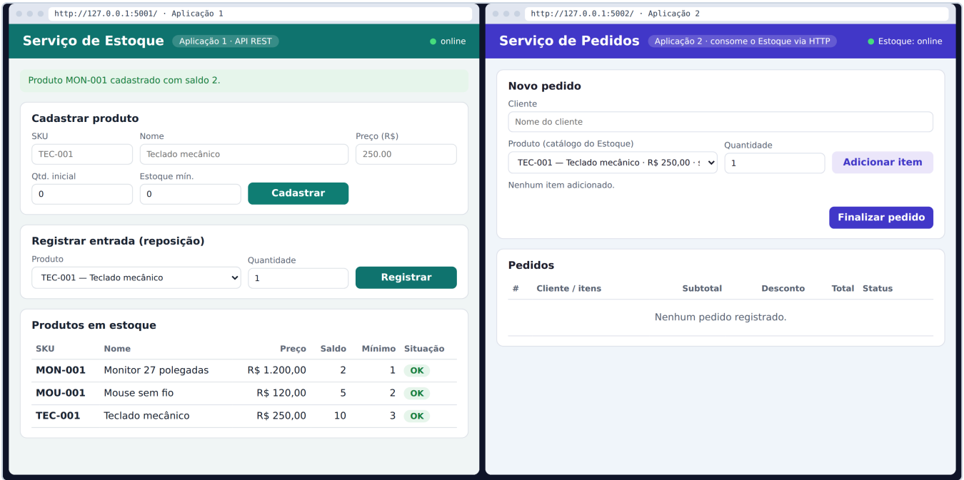
Figura 4: Três produtos cadastrados no Estoque. O catálogo aparece automaticamente no Pedidos.
