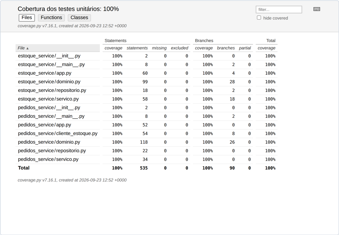
Figura 2: Relatório HTML de cobertura gerado pelo coverage.py (entrega/evidencias/cobertura_html/index.html).
