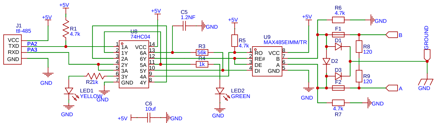
TTL转RS485通讯模块电路（连接太阳能逆变主控）
