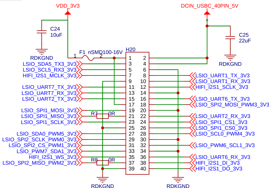
RDK X5开发板40pin输出接口
