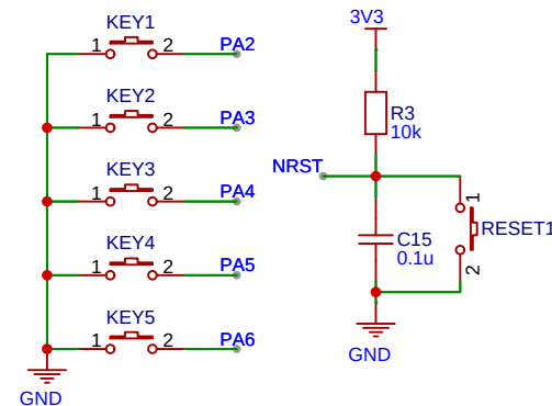
按键电路和复位电路
