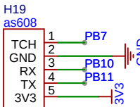
指纹模块接口电路
