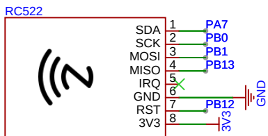
rc522刷卡接口电路
