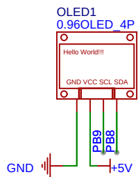
oled显示电路
