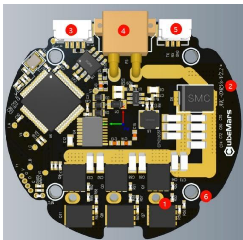
产品规格 (AK-DRV-V2.2 小款)
