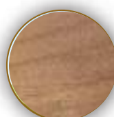
CAMPANO
