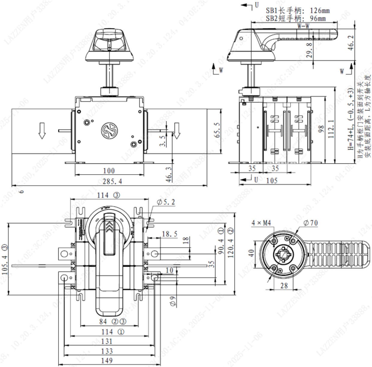
正操外形安装图（分闸）
