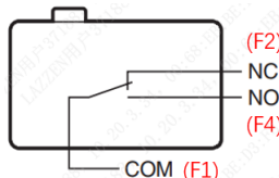
常开+常闭形式(11 形式)
