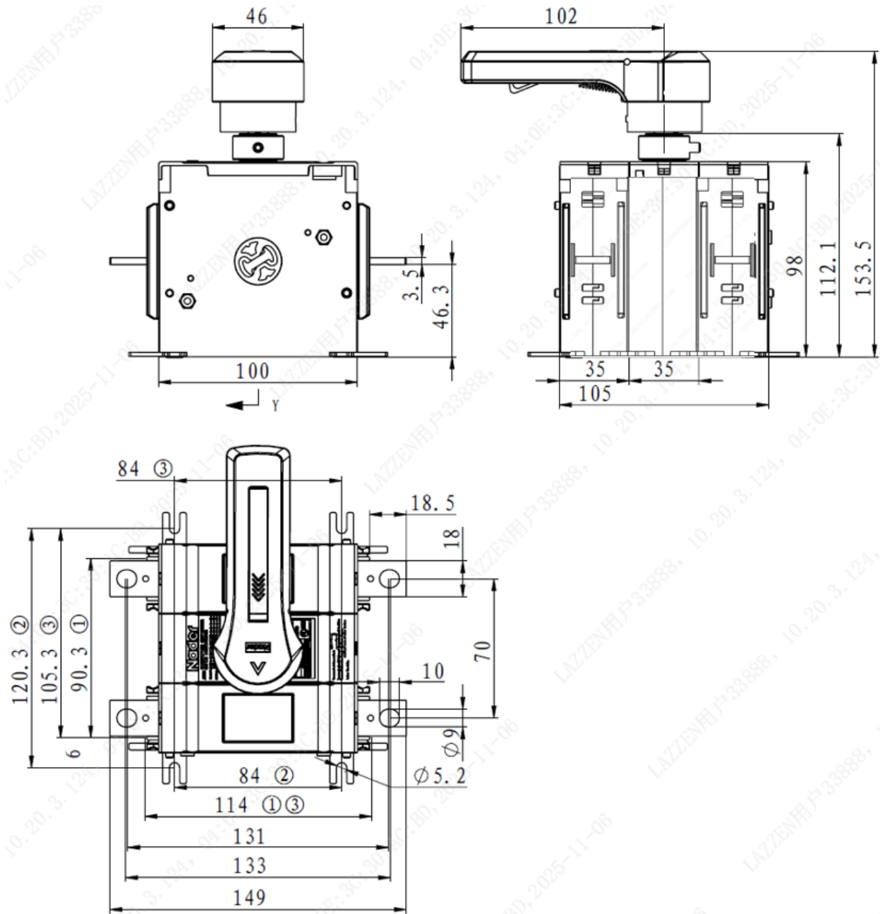
正操（柜内机构居中）外形安装图（分闸）
