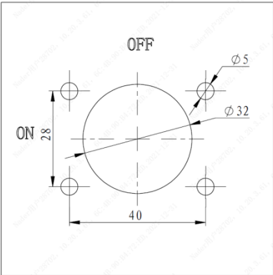
SB 柜外侧操手柄柜门推荐开孔图
