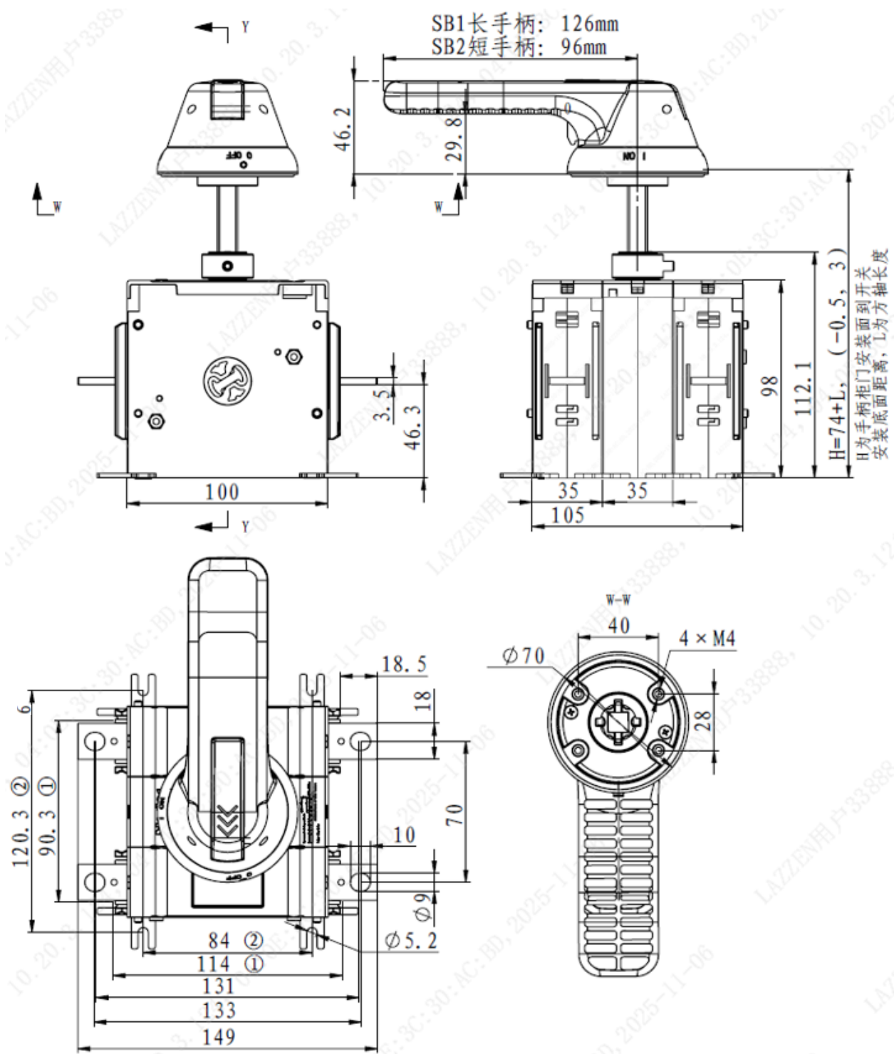
正操（机构居中）外形安装图（分闸）
