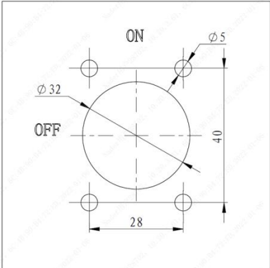
SB 柜外正操手柄柜门推荐开孔图
