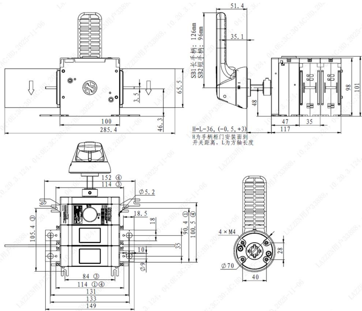
侧操外形安装图（分闸）
