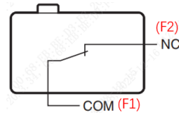
常闭形式(01 形式)
