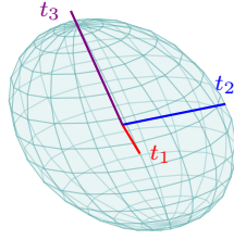
Figure 1: 좌표축과 나란하지 않은 이차곡면과 그 주축 방향 t_1, t_2, t_3 - 세 방향은 서로 직교한다
