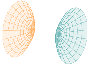
Figure 3: 이엽쌍곡면 – 두 조각으로 분리
