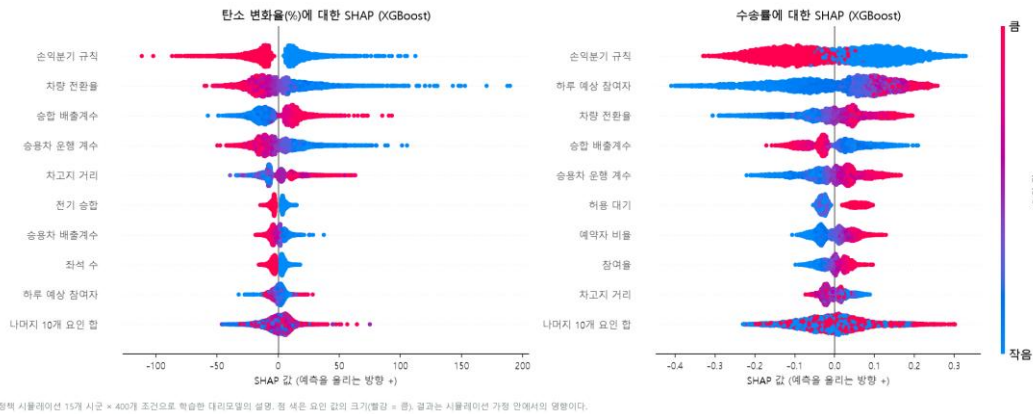
그림 3. 운영 성과 대리모델(XGBoost)의 SHAP 요약: 왼쪽 탄소 변화율, 오른쪽 수송률 (15개 시군 × 400개 조건)
