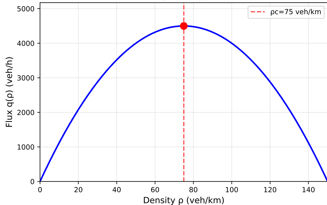
Fundamental Diagram: q(\rho) (Greenshields)
