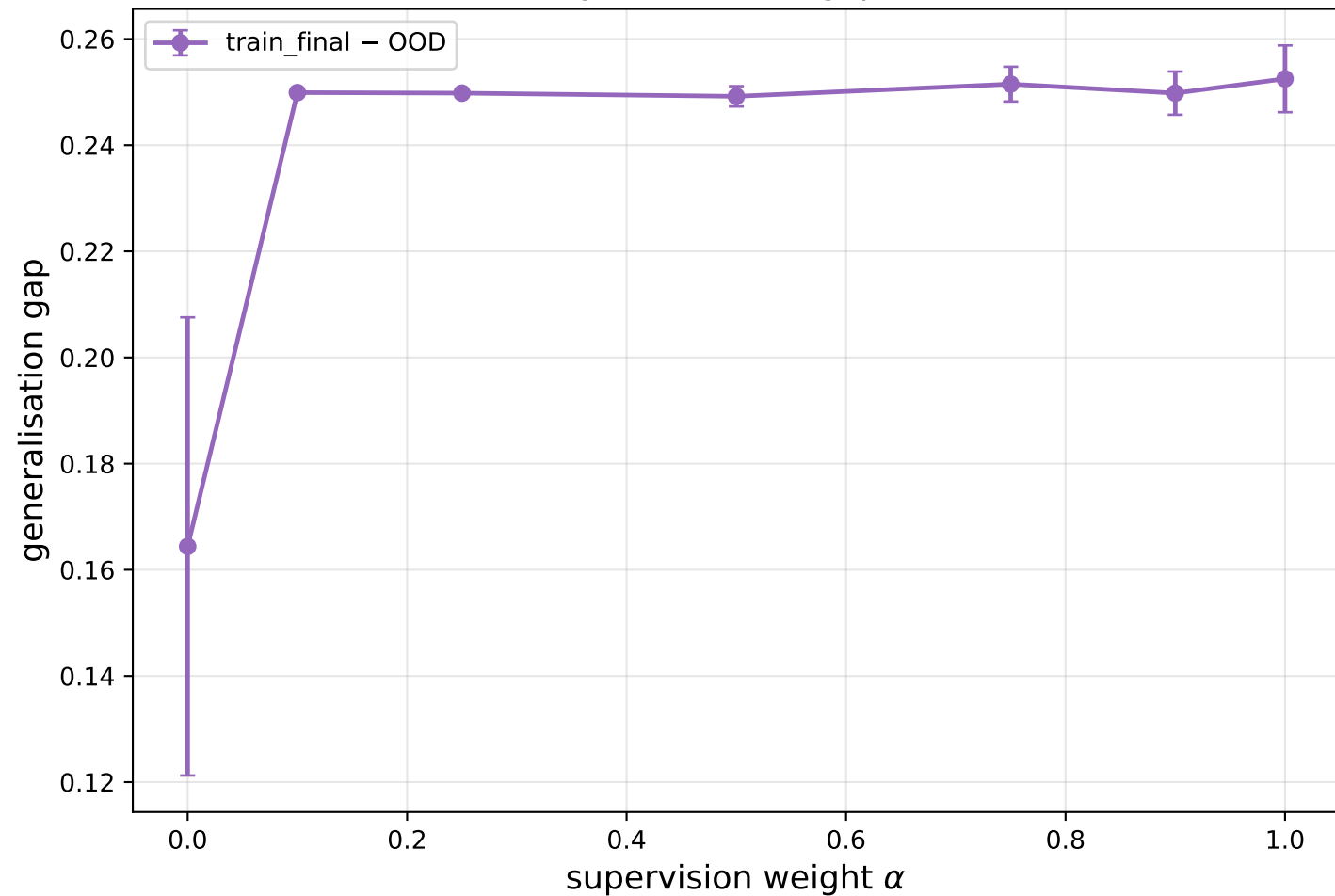
E3: generalisation gap vs \alpha
