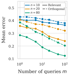
(b) Error vs m
