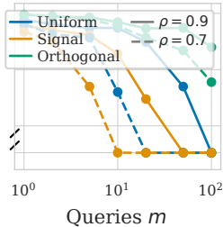
(d) Query distribution n=100, r=5, M=100
