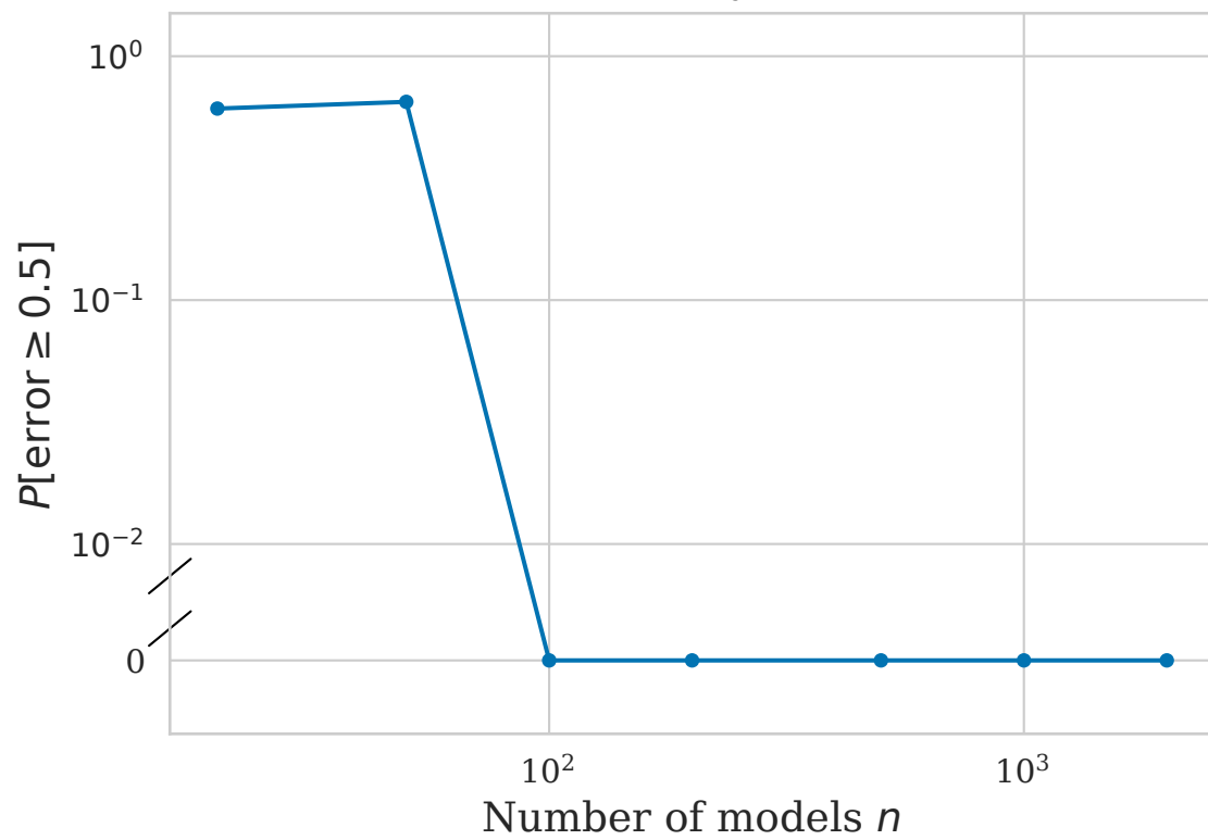
(d) Sample complexity ( r = 5, m = 50 )
