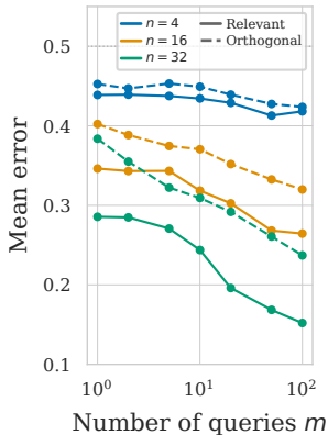
(b) Error vs m
