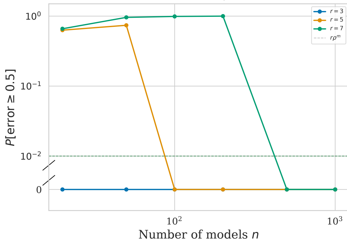
(d) Sample complexity ( m = 50 )
