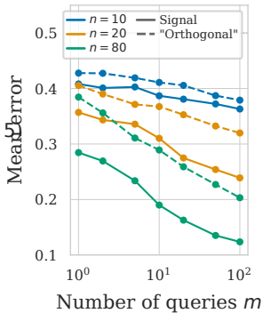
(b) Error vs m
