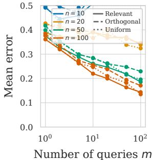
(b) Error vs m
