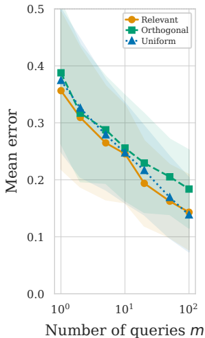
(b) Error vs m
