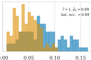
RAG
