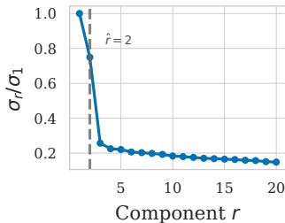
RAG
