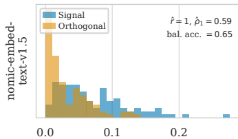
LoRA
