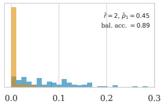
RAG
