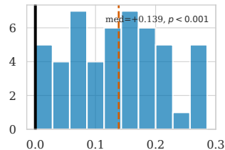
RAG
