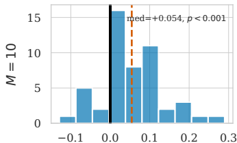
LoRA
