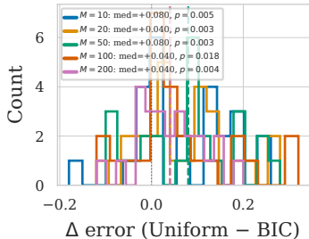
LoRA
