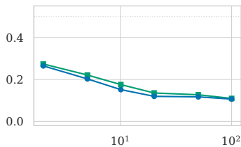
all-MiniLM
