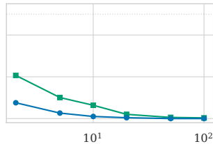
RAG
