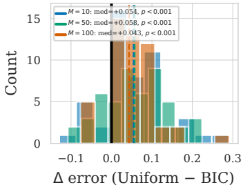
LoRA
