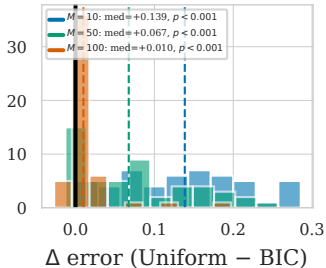
RAG
