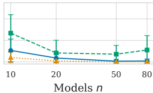
RAG
