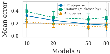
LoRA
