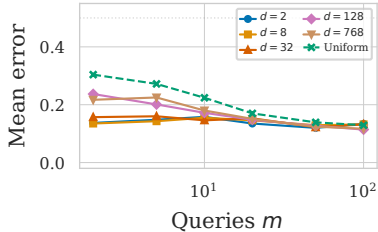
LoRA
