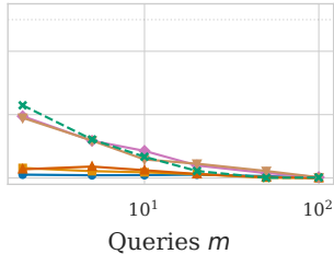
RAG
