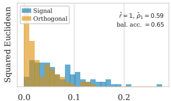
LoRA
