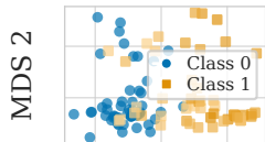
(a) Est. signal queries, m=5
