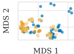
Est. orthogonal queries, m=5
