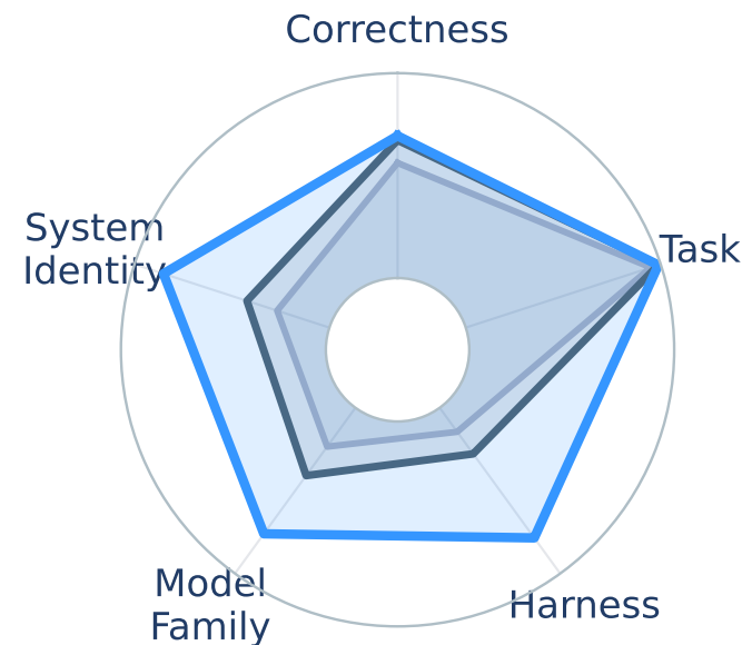
all-mpnet-base-v2
