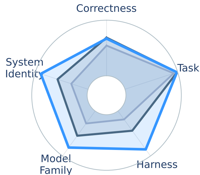
all-mpnet-base-v2
