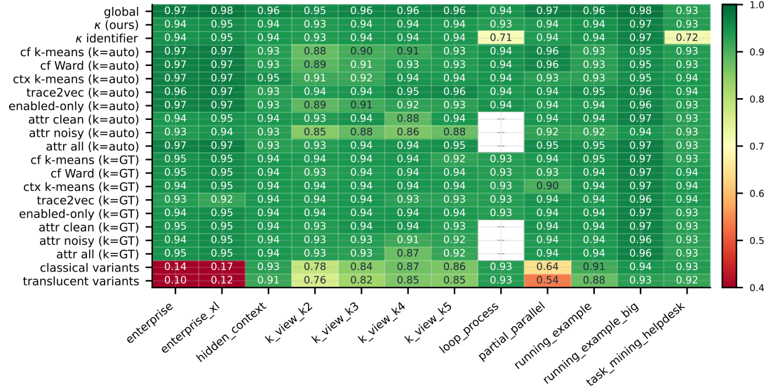
translucent F1
