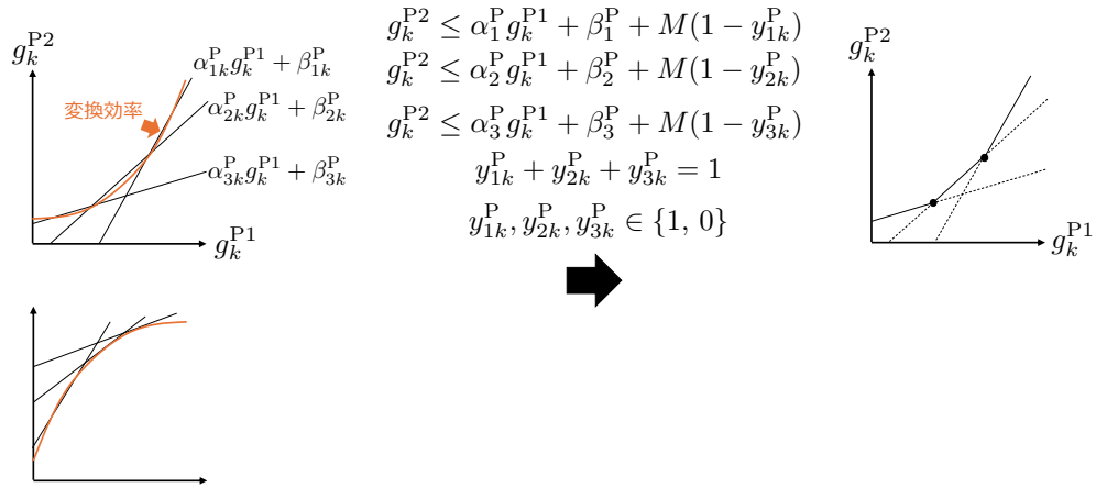
図 3 区分線形関数による表現 (太陽光発電機器の場合)
