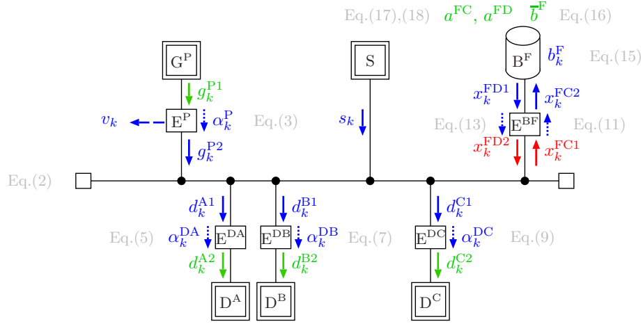
図 2 電力クラスタの構成図 (赤: 決定変数, 青: 従属変数, 緑: 定数 (外生変数))
