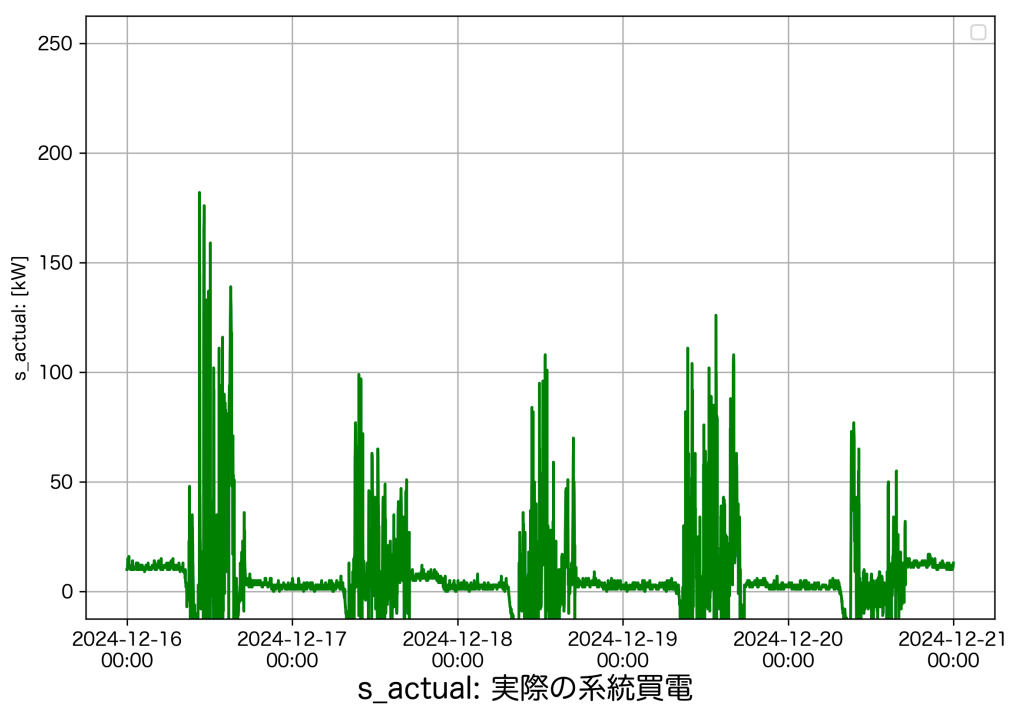
図 10 系統買電の最適化結果と実績値の比較
