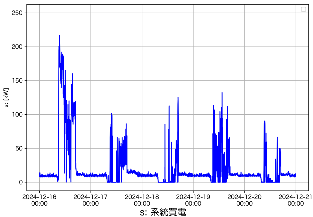
図 8 系統買電（最適化結果）
