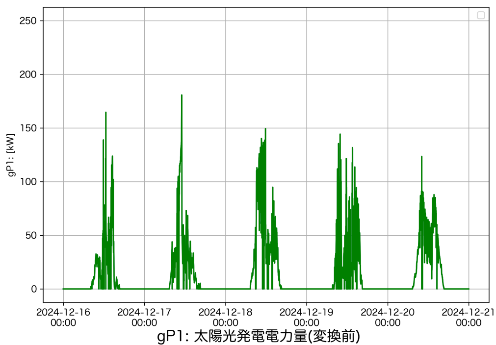
図 4 太陽光発電電力実績データ
