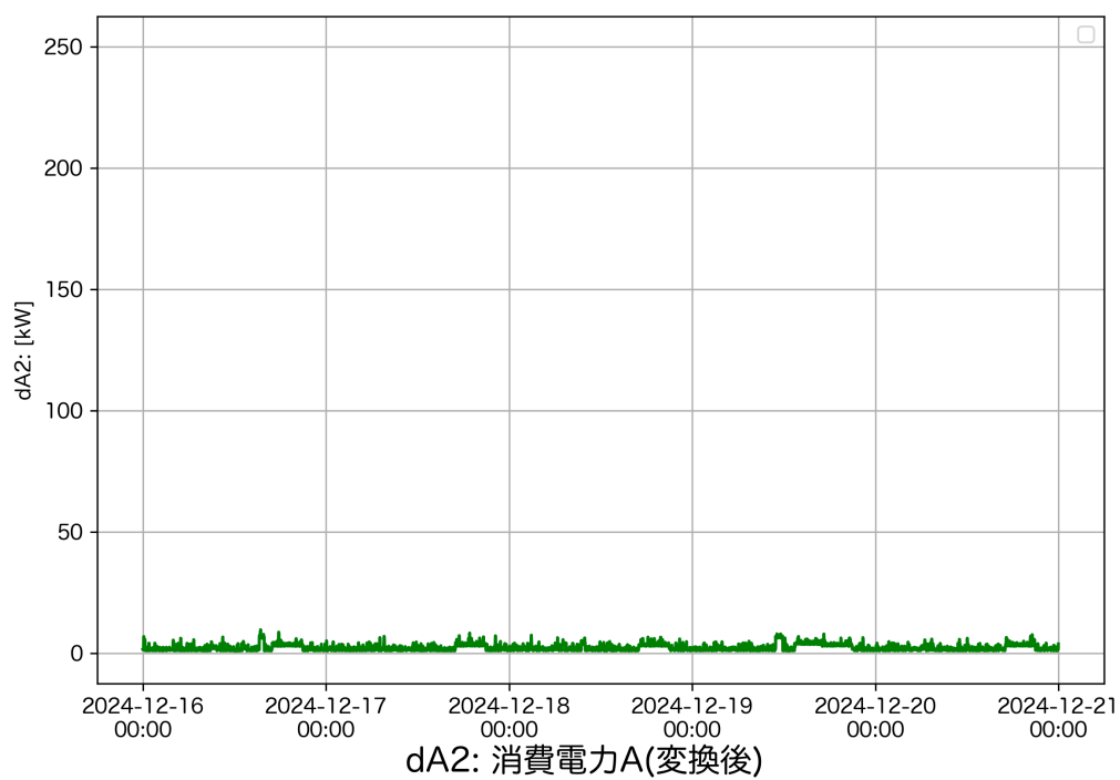
図 5 消費電力 A 実績データ (6600/210-105V 75kVA)
