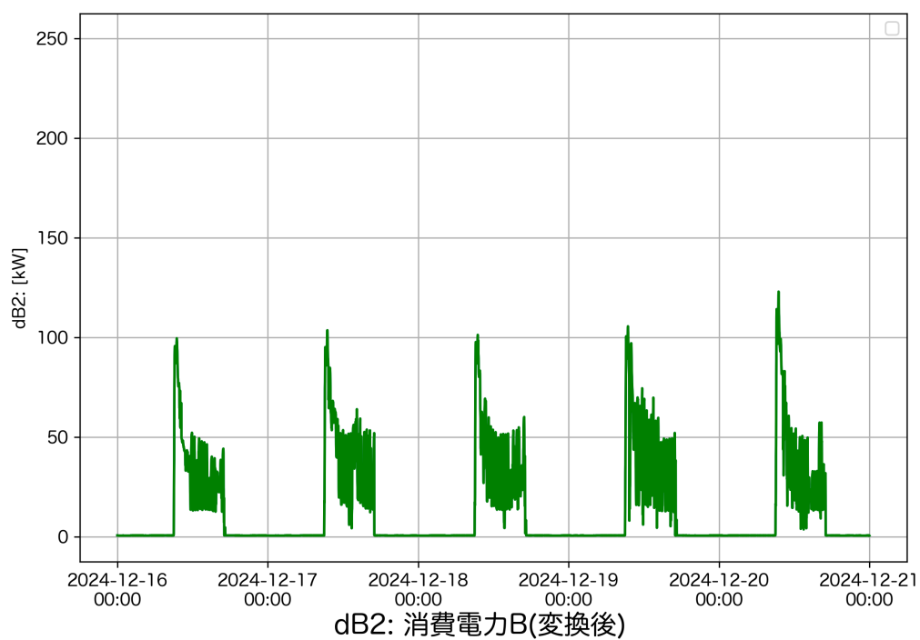
図 6 消費電力 B 実績データ (6600/210V 300kVA)
