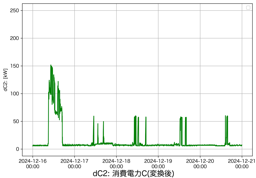
図 7 消費電力 C 実績データ (6600/210V 500kVA)
