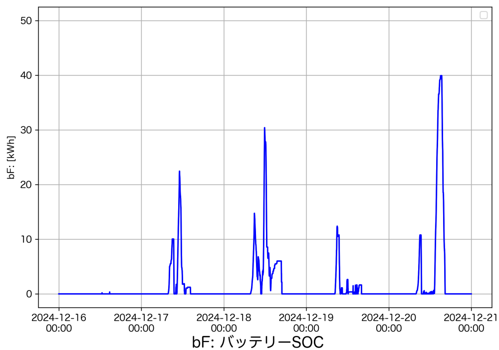
図 9 バッテリー SOC（最適化結果）
