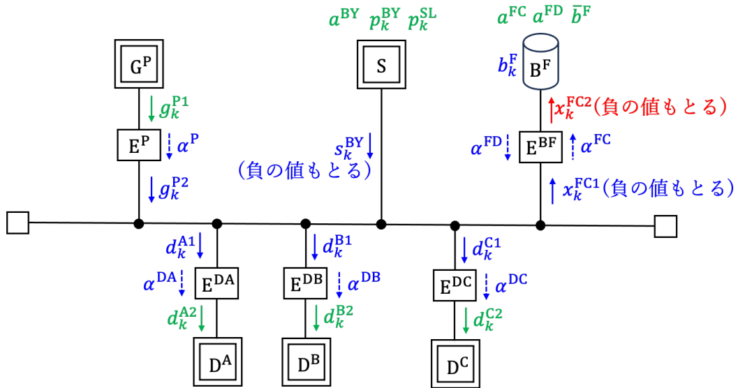
図 2 電力クラスタの構成図 (赤: 決定変数, 青: 従属変数, 緑: 定数 (外生変数))
