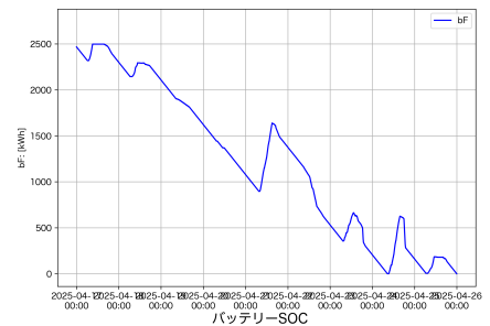
バッテリーSOC
