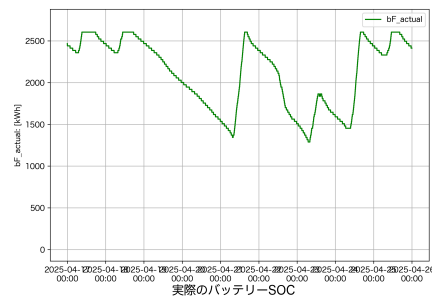
実際のバッテリーSOC
