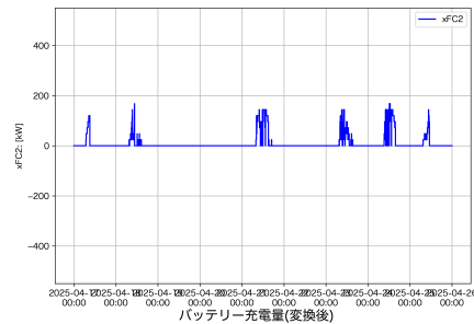
バッテリー充電量(変換後)
