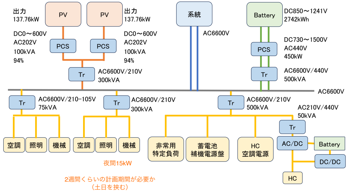
図 1 テクシード構成図
