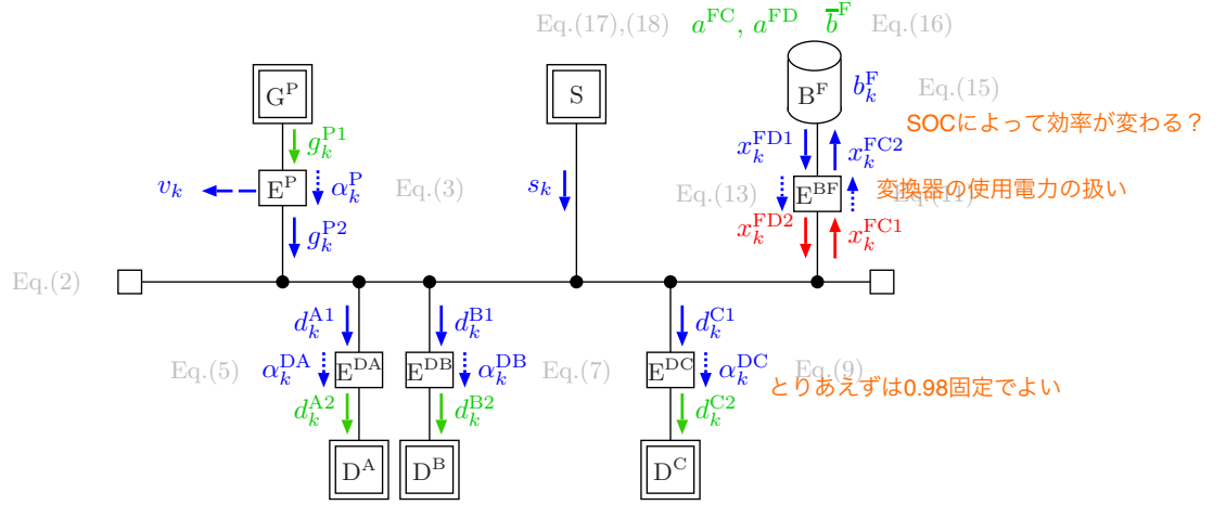
図2 電力クラスタの構成図 (赤: 決定変数, 青: 従属変数, 定数 (外生変数))
