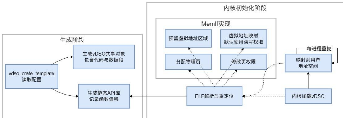
图 3-7 vDSO 生成与映射流程
