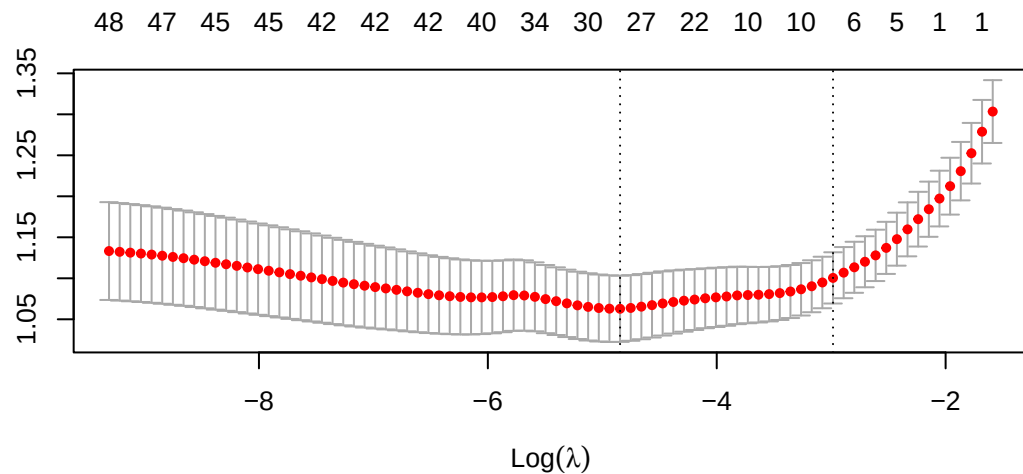
LASSO CV
