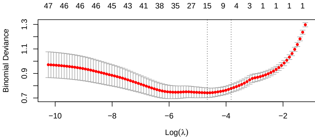
LASSO CV
