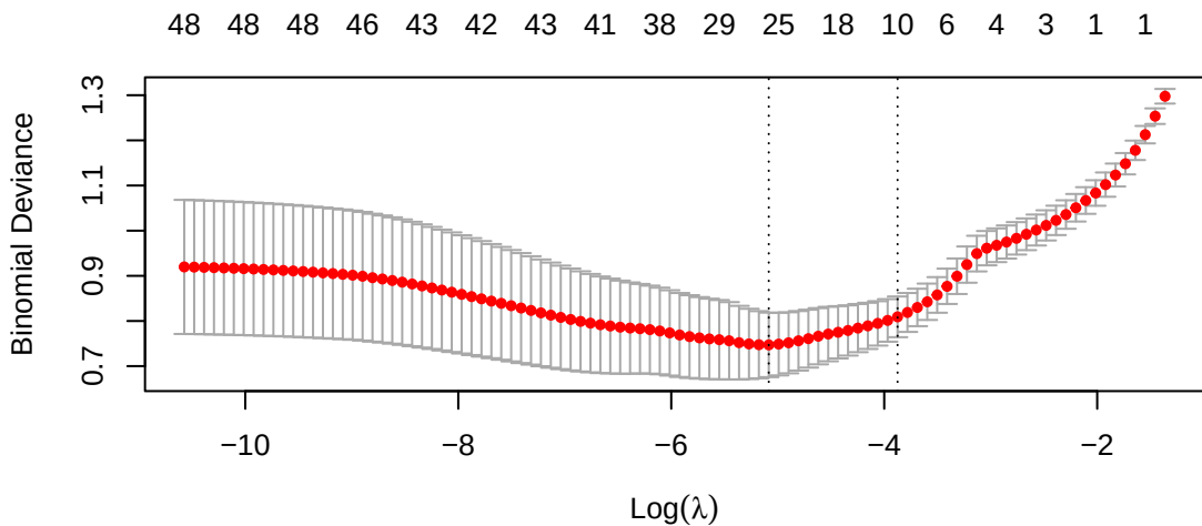
LASSO CV
