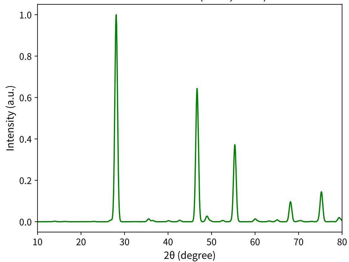
NPT-Berendsen (300K, 1atm)
