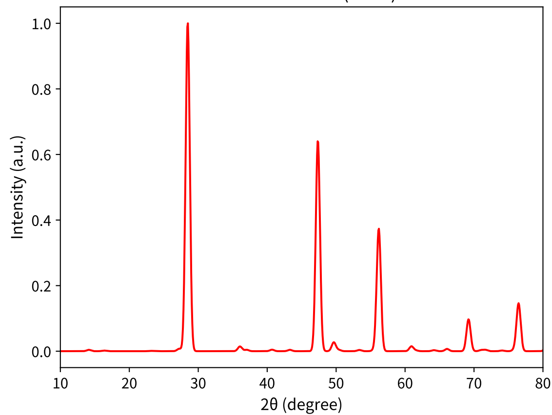
NVT-Berendsen (300K)
