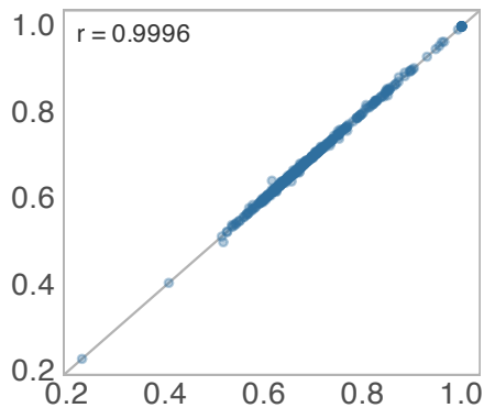
MATTR
