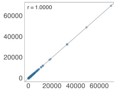
n_char
