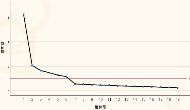
图 6-10 碎石图
