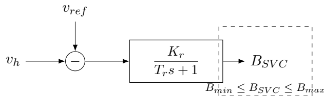
Slika 2.3: SVC Type II - blok dijagram regulatora (prilagođeno prema [?], Fig. 19.3).
