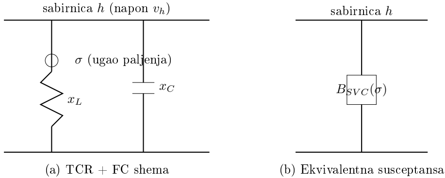
Slika 2.1: SVC shema: (a) TCR + FC konfiguracija, (b) ekvivalentni model preko varijabilne susceptanse B_{SVC}(\sigma) . Prilagođeno prema [?], Fig. 19.1.
