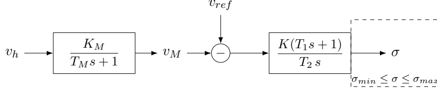
Slika 2.2: SVC Type I - blok dijagram regulatora (prilagođeno prema [?], Fig. 19.2).
