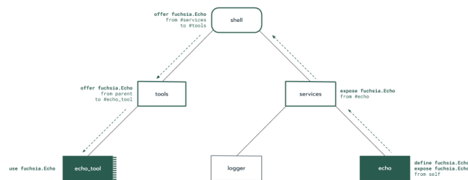
Abbildung 8: Vererbungshierarchie[Goo25]
