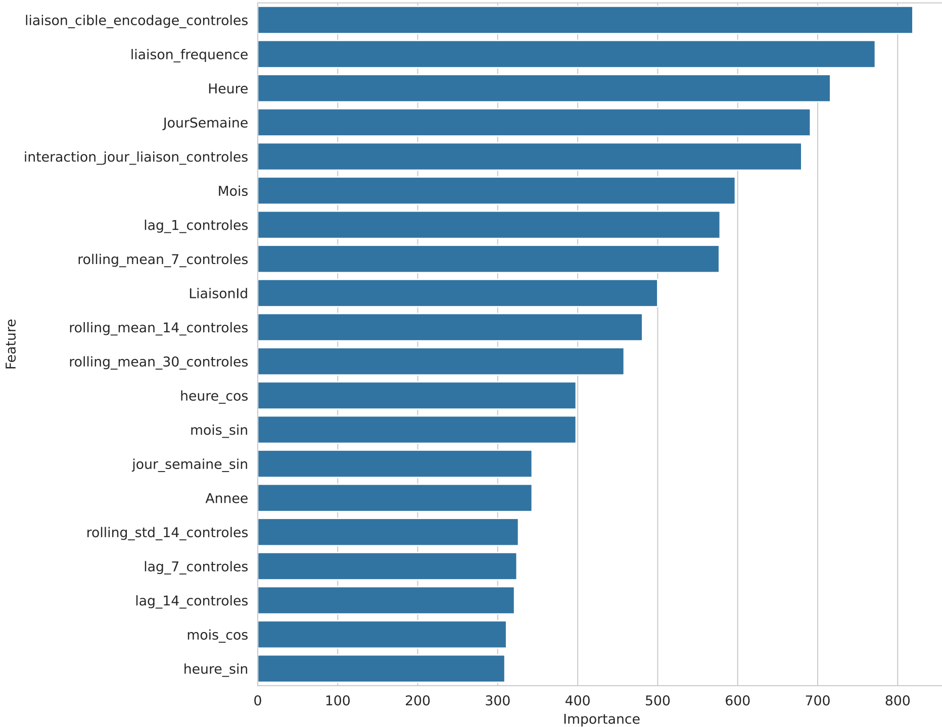
Importance des variables - LightGBM
